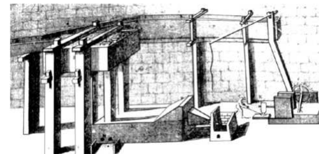
Caixa de vent, forn baix i mall segons Bouchu i Coutrivon (1761)
